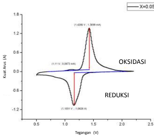
Gambar 16. Grafik CV untuk sampel x = 0.01 diambil pada siklus ke 3.
