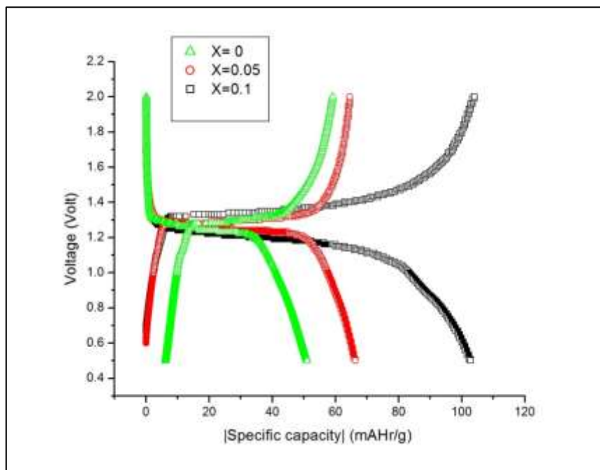
Gambar 18. Grafik charge/discharge pada sampel untuk tiap variasi nilai x .
