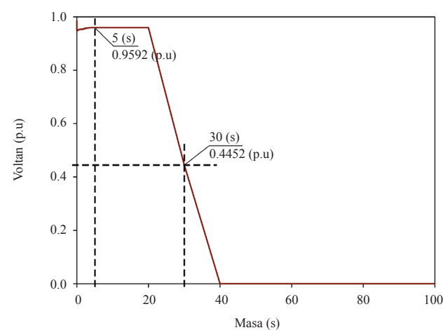
RAJAH 8. Voltan pada Bas 117 ketika putus talian
