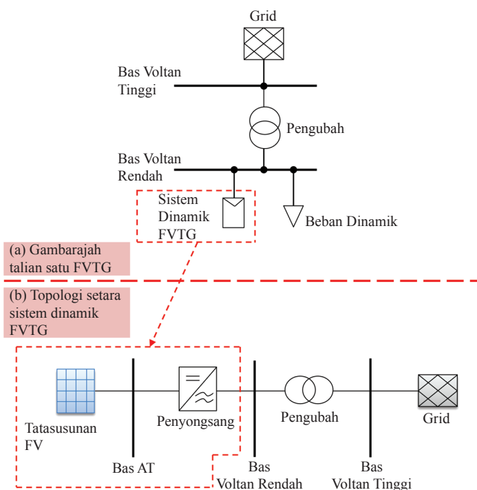
RAJAH 1. (a) Gambarajah talian satu FVTG dan (b) Topologi setara sistem dinamik FVTG Monitor
