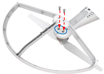
Fig.2 Prop Guard Attachment/图 2 安装桨保护器
