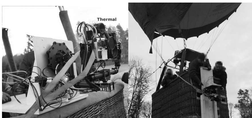
Abb. 1: Aufbau des Kamerakopfes (links) und Anbringung am Ballon (rechts)
