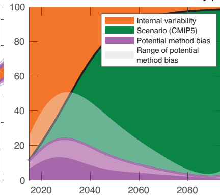
(d) Sahel JJA decadal mean precipitation
