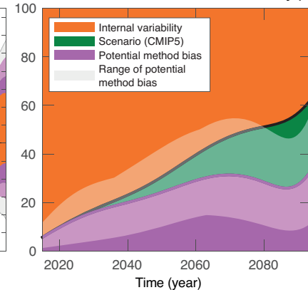
(d) Sahel JJA decadal mean precipitation
