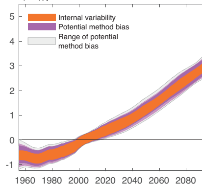
(d) Sahel JJA decadal mean precipitation
