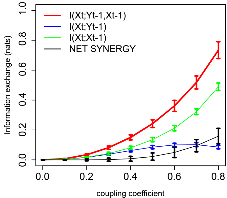
Linear
