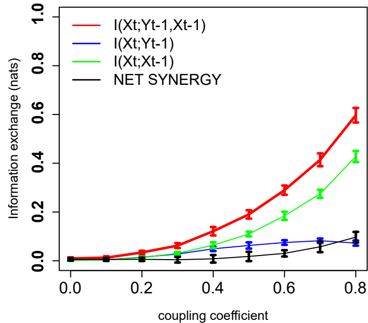
Kernel
