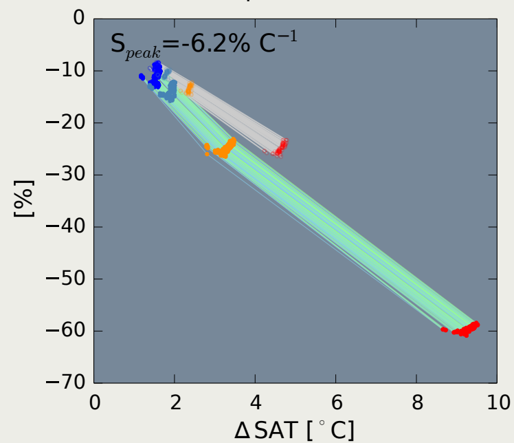
(d) Change in metabolic index (depth < 400 m)
