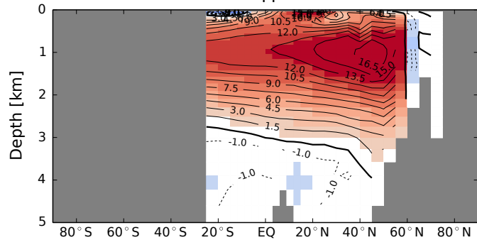
(d) Atlantic meridional overturning [Sv] PI
