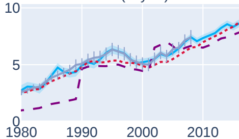
SF6 (kt yr -1 )
