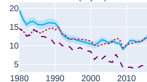
c-C4F8 (kt yr -1 )
