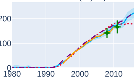
HFC-245fa (kt yr -1 )
