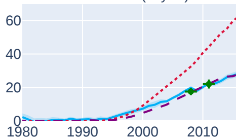
HFC-365mfc (kt yr -1 )
