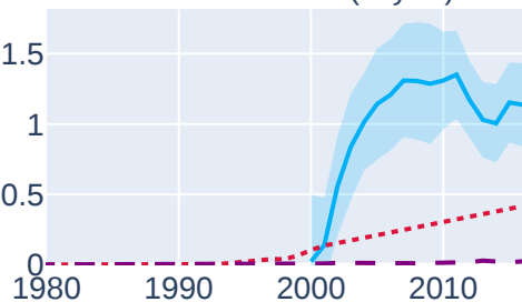
C2F6 (kt yr -1 )
