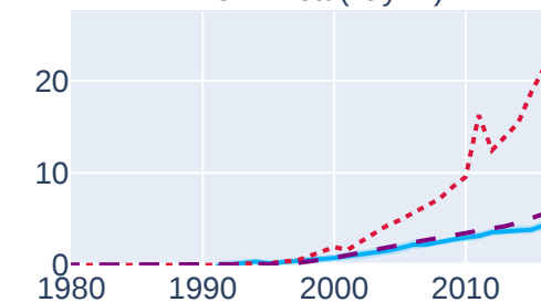
CF4 (kt yr -1 )
