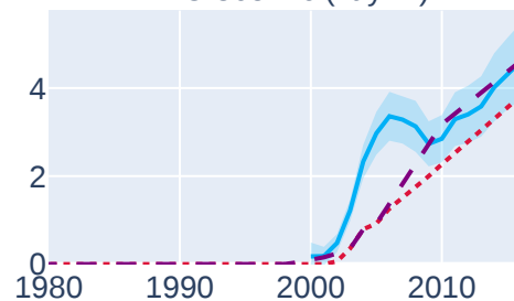
HFC-236fa (kt yr -1 )
