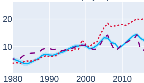
HFC-134a (kt yr -1 )
