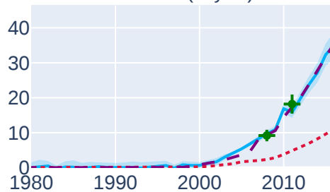
HFC-143a (kt yr -1 )
