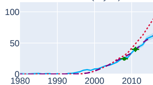
HFC-152a (kt yr -1 )
