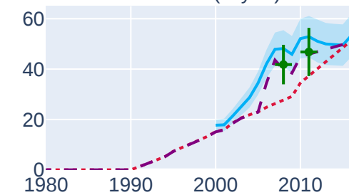
HFC-227ea (kt yr -1 )
