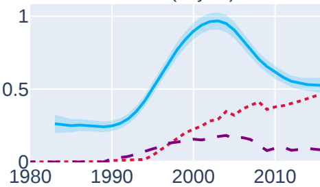
NF3 (kt yr -1 )
