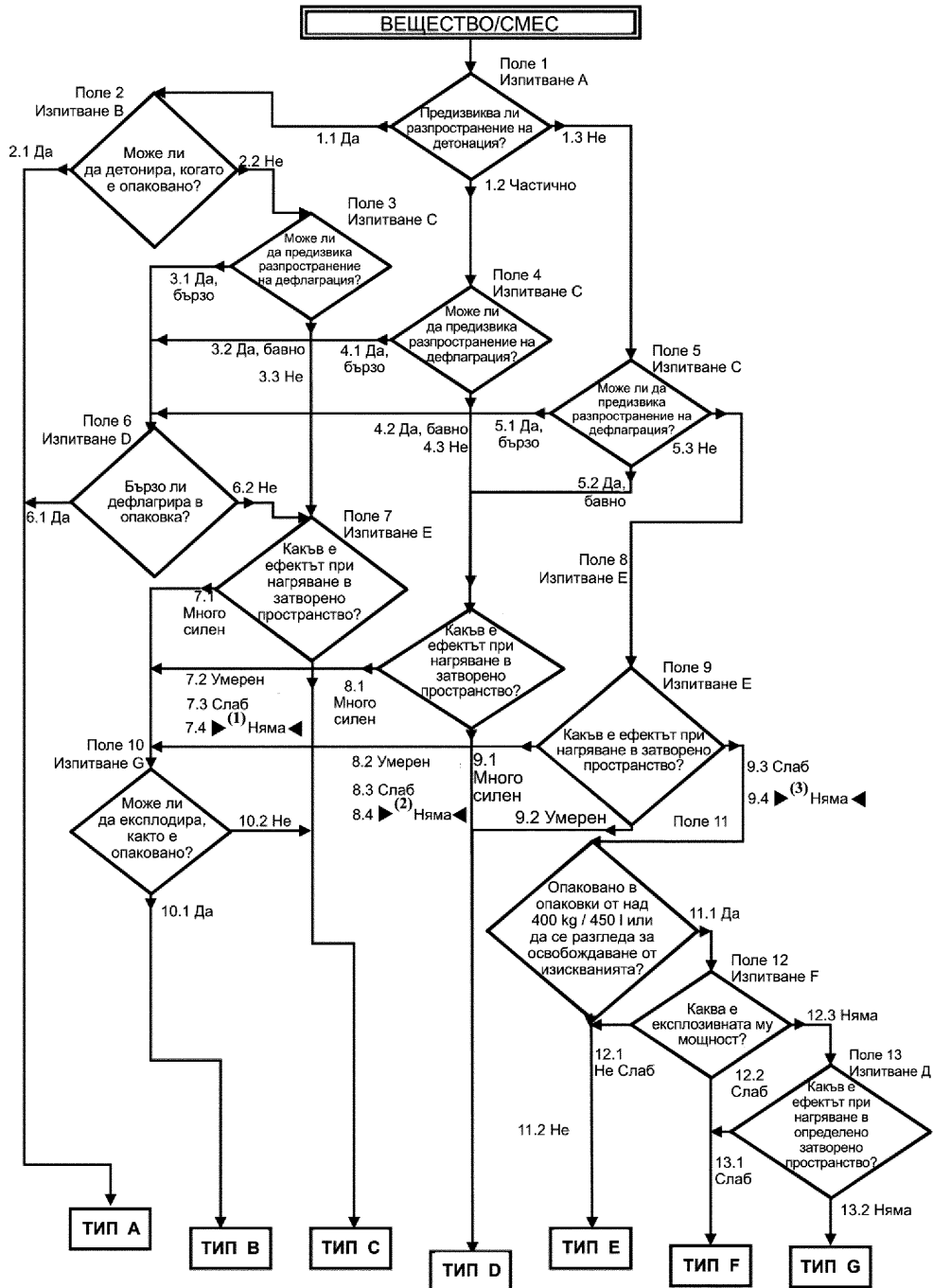
Фигура 2.8.1 Самоактивиращи се вещества и смеси
