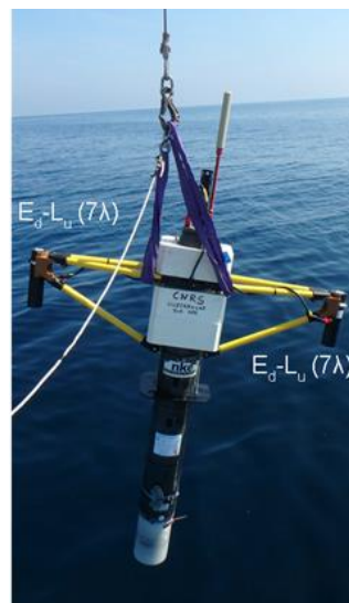
Figure 40: A ProVal float being deployed (N. Mayot).
