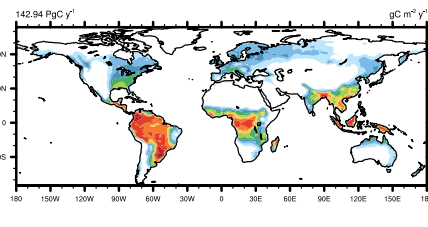
NPP (2000–2013) JULES-C1
