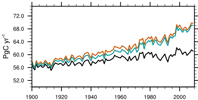
JULES-C2 R_{\text{het}}
