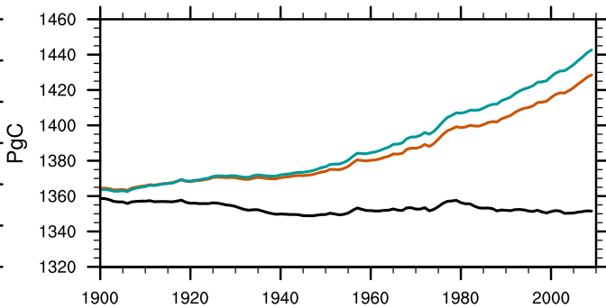
JULES-C2 C_{\text{soil}}
