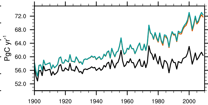
JULES-C2 NBP
