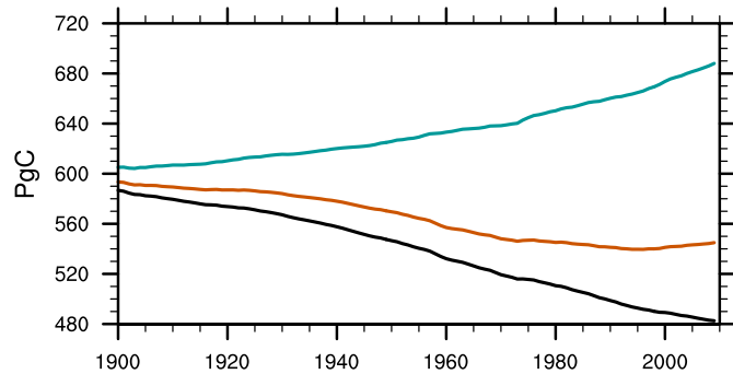
JULES-C2 C_{\text{veg}}
