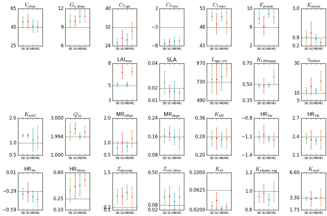
(c) Posterior parameters for TempEBF
