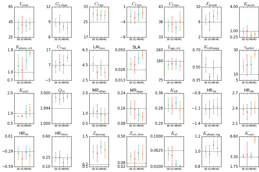
(e) Posterior parameters for BorDBF
