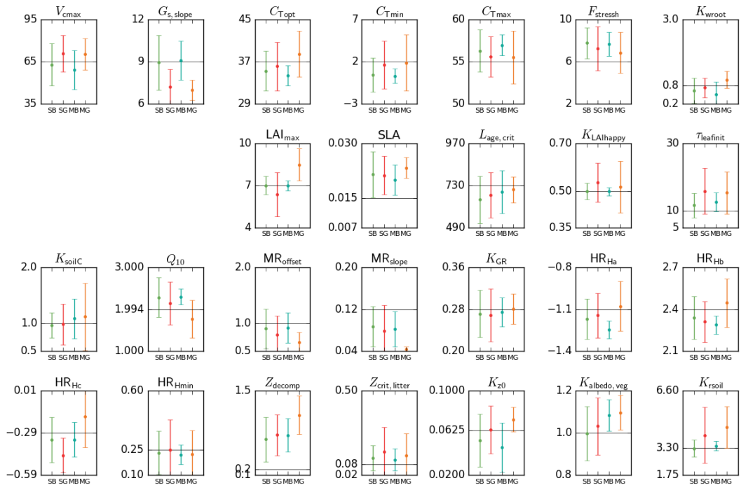
(a) Posterior parameters for TropEBF
