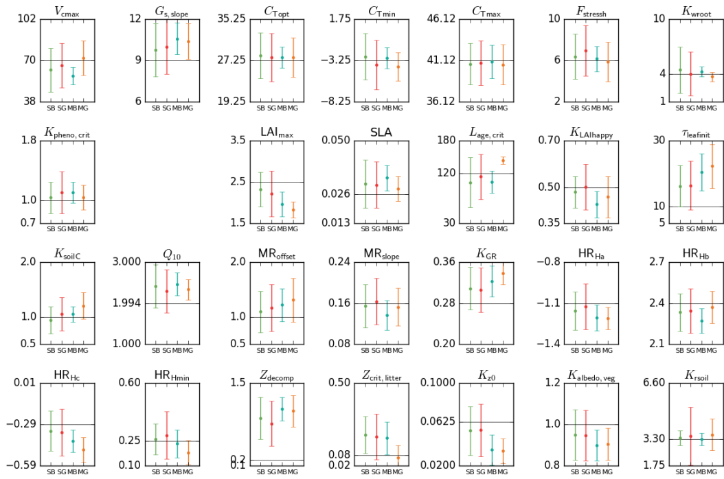
(f) Posterior parameters for C3grass
