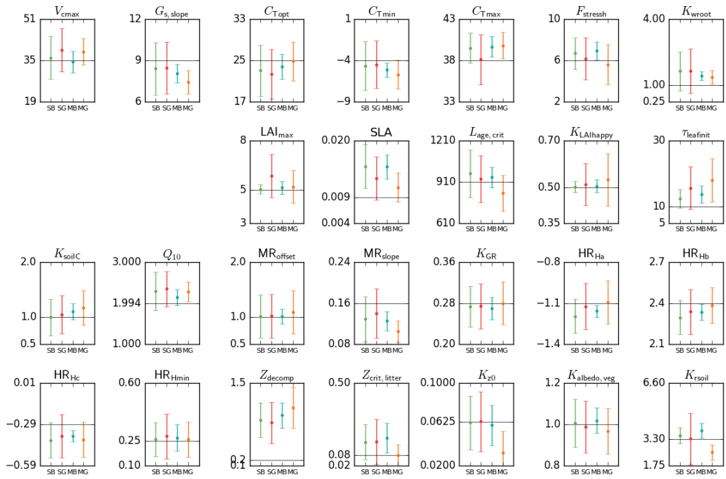
(b) Posterior parameters for TempENF
