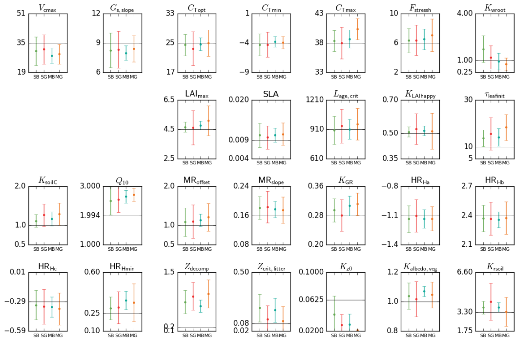
(d) Posterior parameters for BorENF
