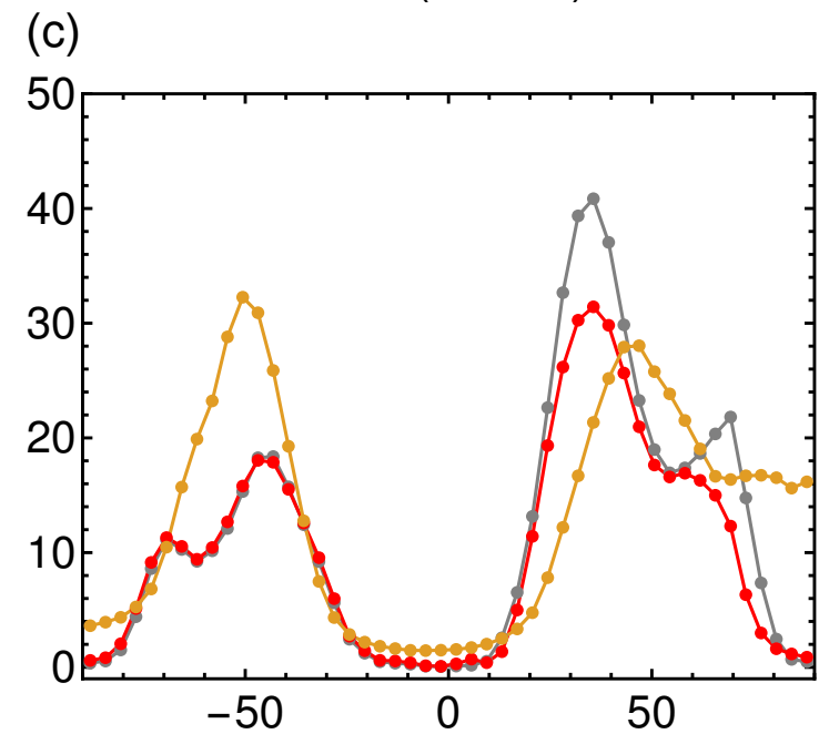
La Niña (500 mb)
