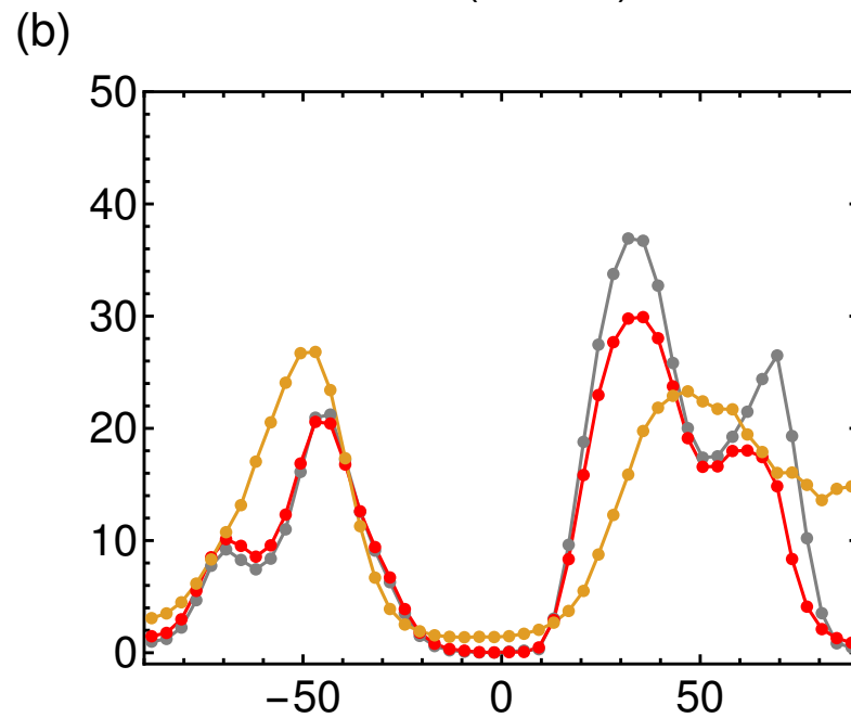
El Niño (500 mb)
