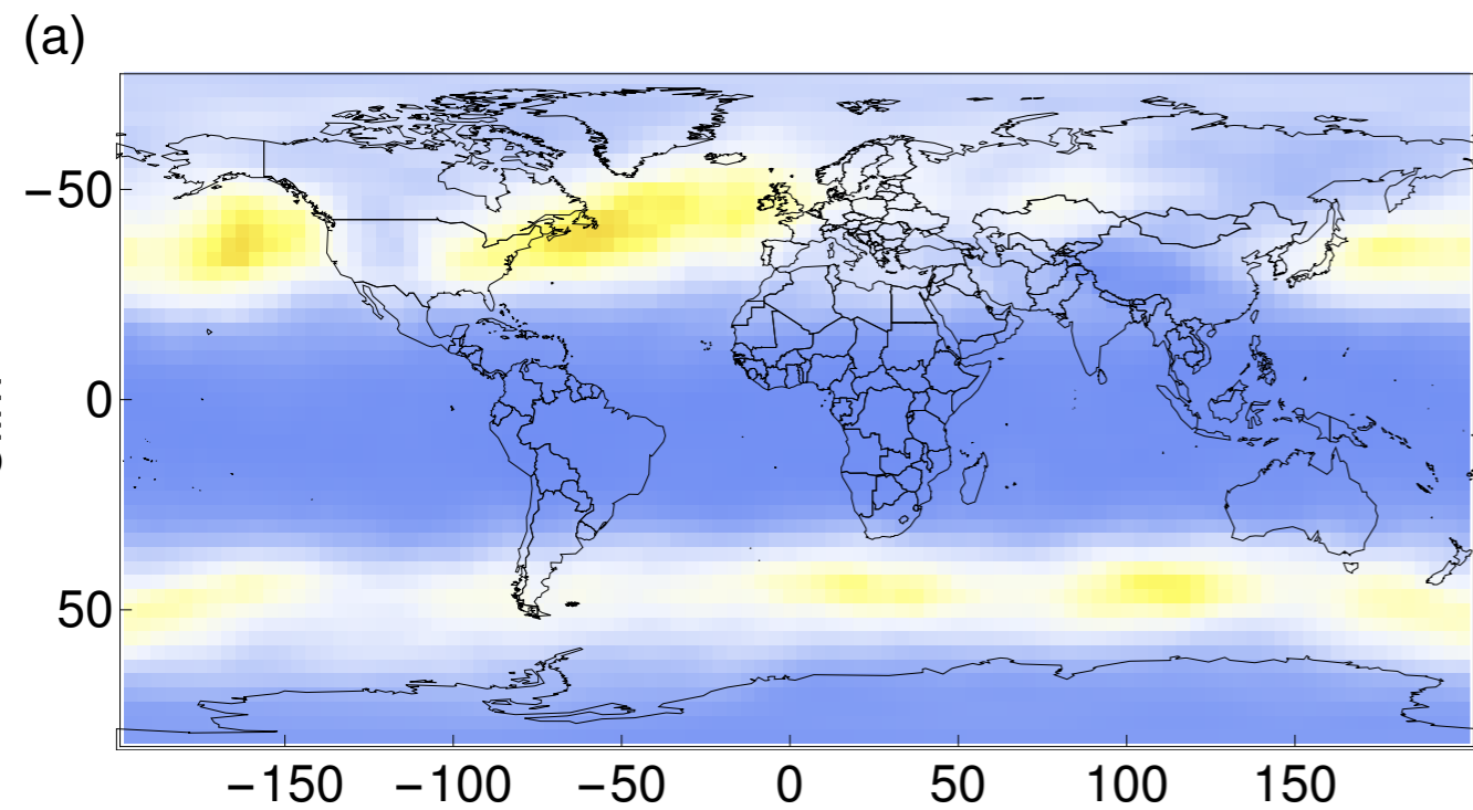
ERA-Interim EKE (500 mb)
