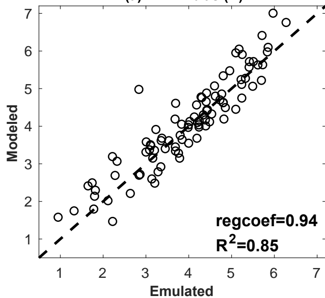
(d) JJAT bias (C)
