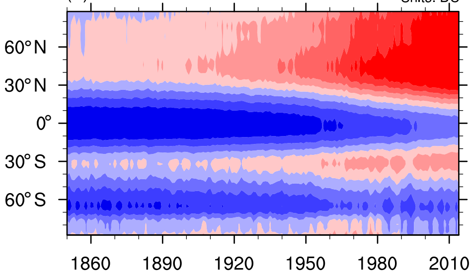
(a) BCC-ESM1
