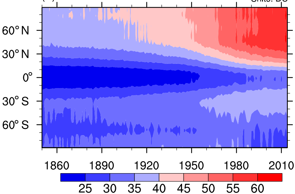
(b) CMIP6
