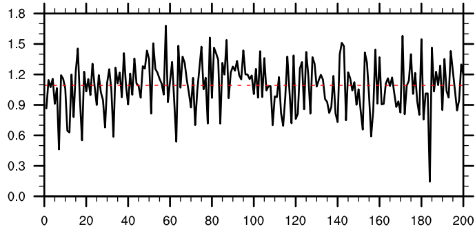
(d) NH and SH sea ice extent ( \times 10^6 \text{ km}^2 )
