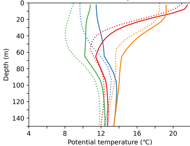
(d) Mid-Atlantic Bight EPU
