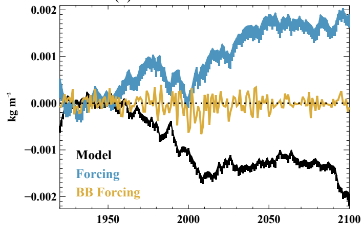
(d) Attribution Global \Delta LWP
