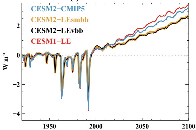
(e) Global \Delta FSNTC
