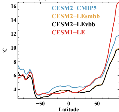
(d) Attribution 2080–2100 \Delta SAT
