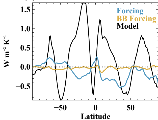
(d) Attribution 2080–2100 CldFB
