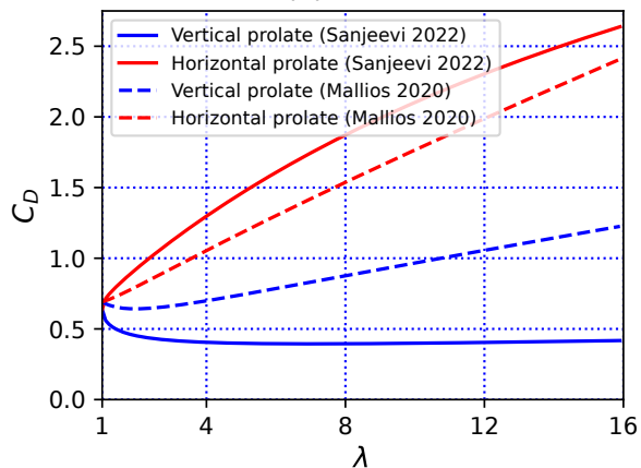
(d) Re = 300
