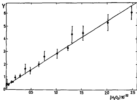
Рис. 1. Вид функции Y([H_2O_2]) и экспериментальные значения.
