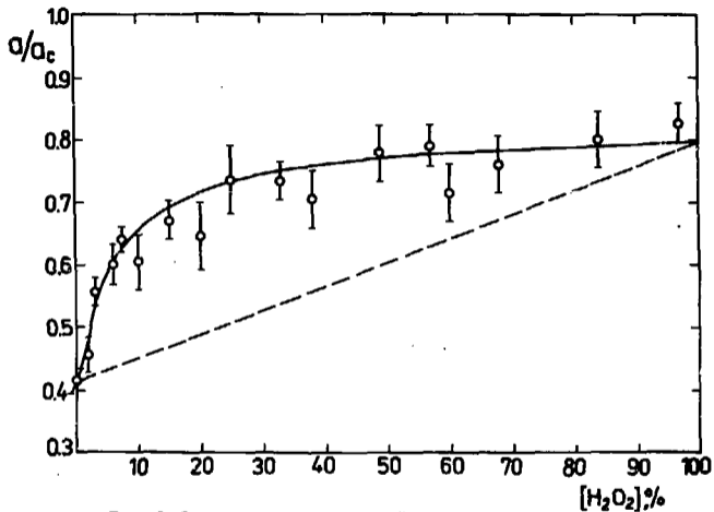
Рис. 2. Зависимость остаточной поляризации отрицательных мюонов от концентрации водного раствора перекиси водорода.
