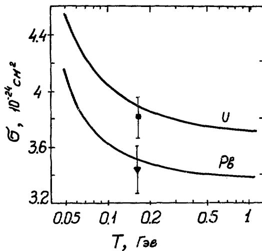
Рис. 1. Сечение неупругого взаимодействия дейтронов с ядрами свинца и урана. Указаны экспериментальные точки из работы 19) .
