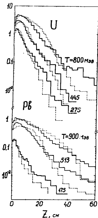
Рис. 4. Распределение плотности нейтронов W(z) = 2\pi \int W(z, r) r dr вдоль оси урановой и свинцовой цилиндрических мишеней с диаметром 10 и длиной 60 см, облучаемых протонами /пунктир/ и дейтронами /сплошные гистограммы/. Указаны энергии первичных частиц / в МэВ ах/. Значения W(z) даны в расчете на одну первичную частицу.
