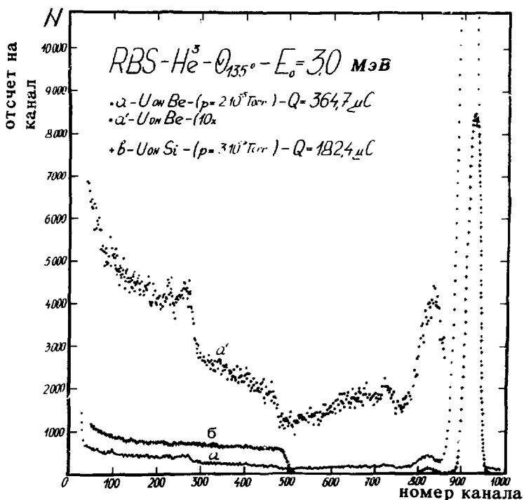
Рис. 3. Энергетический спектр рассеянных частиц ^3\text{He} от пленок урана на подложках из бериллия и кремния.
