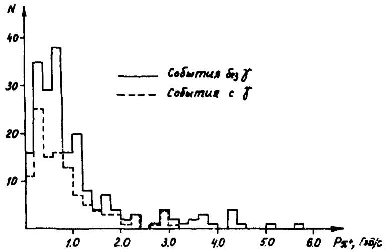
Спектр импульсов \pi^+ -мезонов.
