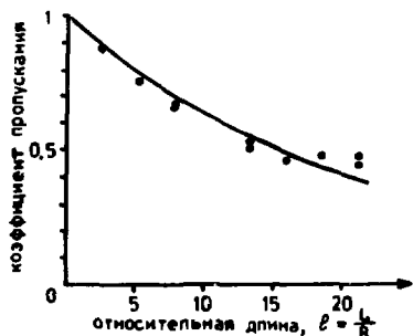
Рис.3. Сравнение расчета с экспериментом.
