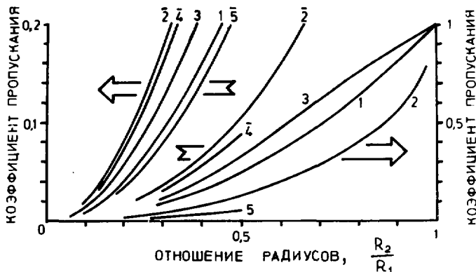
Рис.2. Пропускание света различными световодами.
