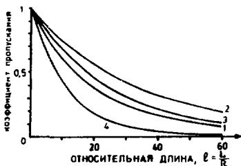
Рис.1. Пропускание света цилиндрической частью счетчиков.
