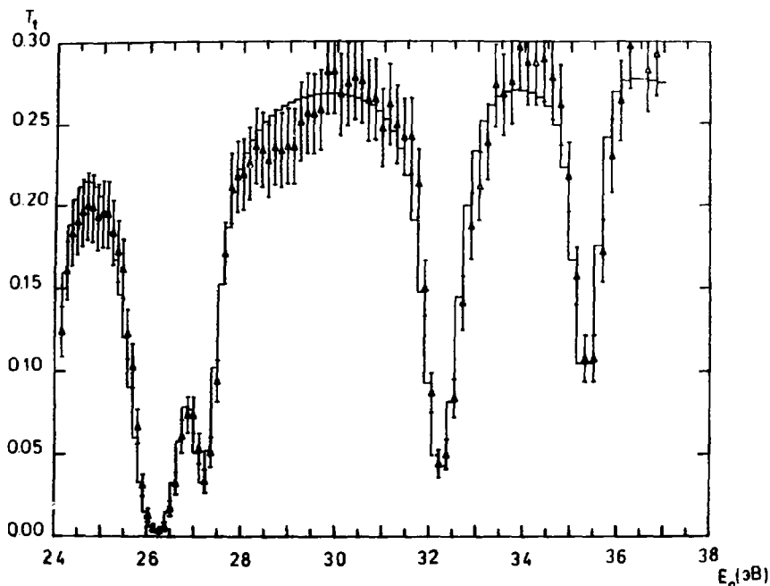
Рис.1. Результат многоуровневой параметризации функции пропускания при толщине образца 0,1234 яд./барн. \Delta - экспериментальные значения с ошибками, непрерывная кривая - восстановление величины пропускания по полученным параметрам.
