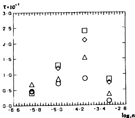
Рис. 2. Зависимость величины \tau от логарифма толщины образца /яд./барн/ для резонансов с энергиями: \circ - 26, 27 эВ; \Delta - 27, 26 эВ, - 32, 30 эВ, \square - 35, 39 эВ.
