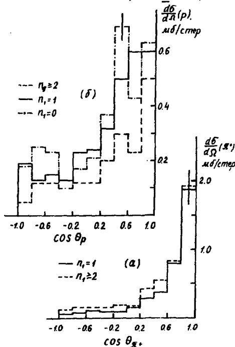
Рис.1. Распределение d\delta/d\Omega в зависимости от косинуса угла вылета \pi^+ -мезонов/а/ и протонов /б/.
