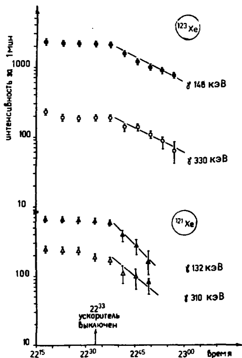
Рис. 4. Спад активности ^{121}\text{Xe} и ^{123}\text{Xe} после окончания облучения \text{SvCl} .
