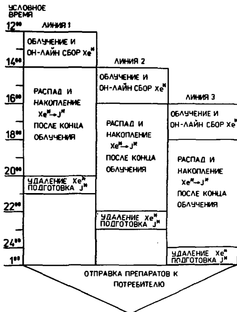
Рис.2. Схема он-лайн процесса получения ^{123}J из ^{123}He в одном сеансе работы на ускорителе.
