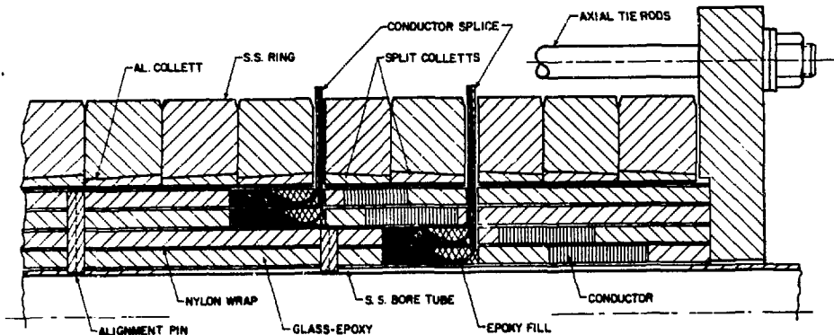
LONGITUDINAL CROSS SECTION OF 4 LAYER DIPOLE D-9A
