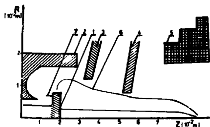
Рис.2. Схема запирающей электромагнитной системы: обозначения 1-6 имеют тот же смысл, что и на рис.1, 7 - траектория электрона в случае запираения.
