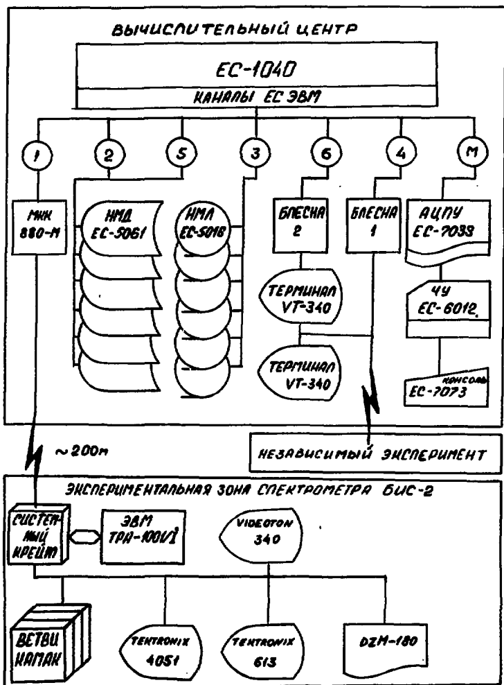
Структура распределенной вычислительной системы.
