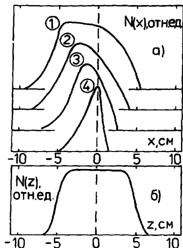
Рис. 3. а) Форма распределения N(x) при Z_{и} = 68 мм и \phi = \psi = \pm 15^\circ для разных значений X_{и} (1 - 68 мм, 2 - 45 мм, 3 - 23 мм, 4 - 0 мм); x отсчитывается от точки пересечения плоскости изображения центральной траекторией в медианной плоскости (см. рис. 1). б) Форма распределения N(z) при Z_{и} = 68 мм; z отсчитывается от точки пересечения центральной траекторией плоскости изображения в направлении, перпендикулярном медианной плоскости (см. рис. 1).
