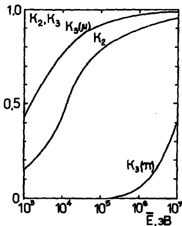
Рис. 6. Зависимость параметров K_2 и K_3 от E .
