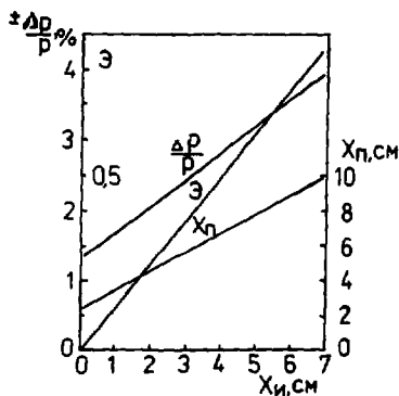
Рис. 5. Зависимость параметров \mathcal{E} , \pm \Delta p/p и X_n от X_n .
