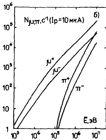
Рис. 8. Зависимость интенсивности мюонов и пионов от энергии для мюонных пучков с примесями: а) для лаборатории №4 и б) для низкофоновой лаборатории.
