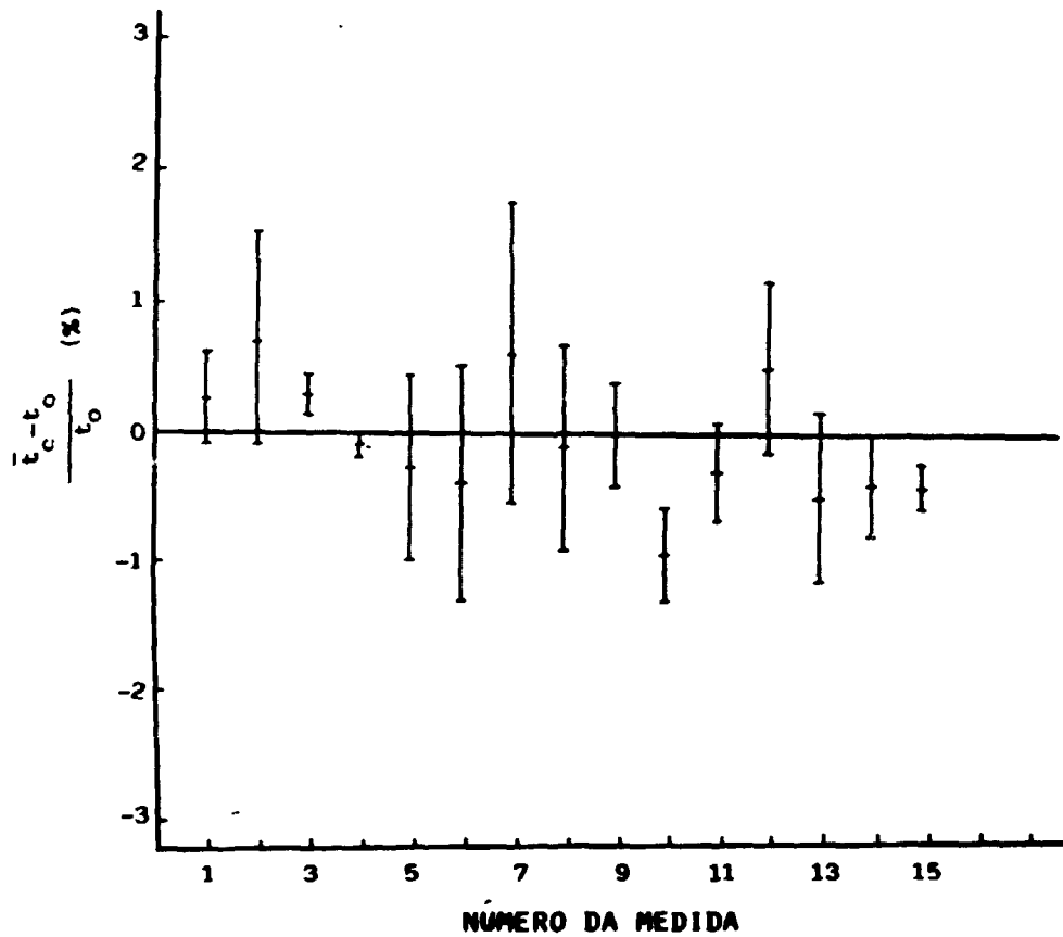
Fig. 1 : Teste de estabilidade a longo prazo da câmara construída, utilizando a fonte de ^{90}\text{Sr} (0,3mCi). Cada ponto representa o valor médio de onze leituras.
