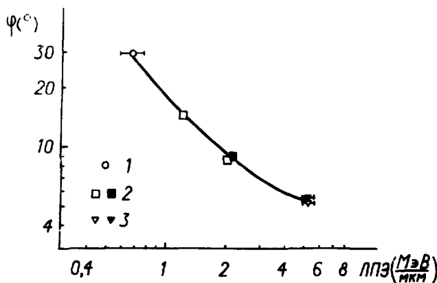
Рис. 2. Средний угол раствора конуса каналов пор в III-мембранах как функция линейной передачи энергии /ЛПЭ/ ускоренных ионов азота /1/, аргона /2/ и ксенона /3/ при фиксированных условиях химической обработки, ЛПЭ рассчитана по методике 19/ . Светлые и темные символы относятся к данным экспериментов с пленками I и II соответственно.
