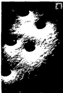
Рис. 1. Электронные микрофотографии ядерных мембран на основе III-пленок, облученных ионами ксенона с полной энергией 125 МэВ. Плотность пор 10^7 \text{ см}^{-2} : а/ мембрана на основе пленки I. Увеличение 9300. Вертикальная и горизонтальная
