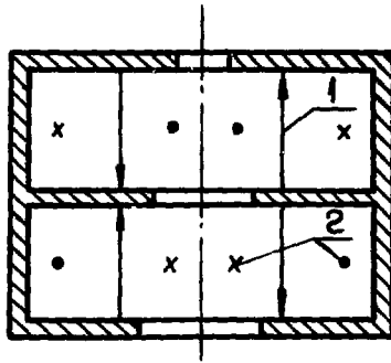
Рис.1. Два связанных E_{110} резонатора, \nabla - вид; 1 - линии электрического поля 2 - линии магнитного поля
