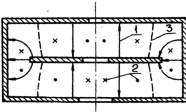
Рис.2. Двухззорный резонатор с шайбой, резонанс "Квази E_{120} "; 1 - линии электрического поля 2 - линии магнитного поля 3 - линия E = 0
