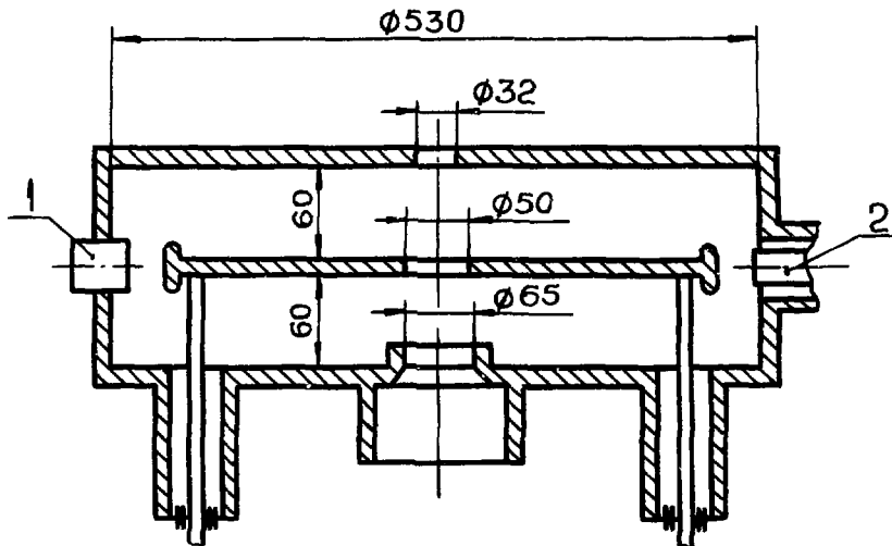
Рис.4. Конструктивная схема резонатора развертки на частоту 915 МГц (тип "Квази E_{120} "); 1 - элемент подстройки частоты, 2 - элемент связи с генератором (шайба гальванически развязана от корпуса резонатора, чтобы обеспечить возможность подавления мультипактора путем подачи постоянного напряжения) .
