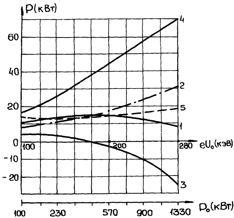
Рис.3. Расчетная ВЧ-мощность для угла отклонения \alpha = 11,5^\circ (0,2 радиана). Шкала мощностей P_0 = F(eU_0) соответствует электронооптической системе, рассмотренной в [2]. Зависимость от энергии приведена для резонаторов, зазор которых оптимизирован при eU_0 = 250 кэВ, f = 915 МГц. 1 - Мощность ВЧ генератора для двухзазорного резонатора с шайбой. 2 - Тепловые потери в стенках резонатора с шайбой. 3 - Мощность ВЧ взаимодействия с пучком в резонаторе с шайбой. 4 - Мощность ВЧ генератора для оптимизированного однозазорного резонатора [1]. 5 - Мощность тепловых потерь в однозазорном резонаторе с углом пролета (для энергии eU_0 = 250 кэВ) [3].
