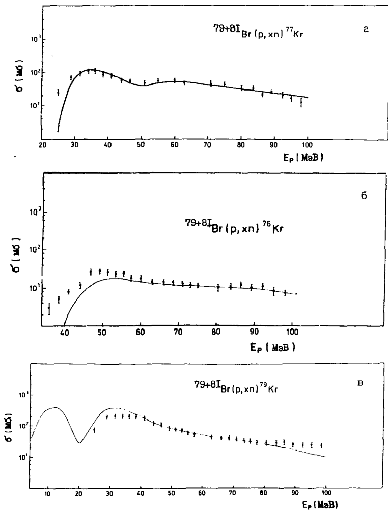
Рис. 3. Измеренные (точки) и рассчитанные (кривые) функции возбуждения реакций: а) \text{прир. Br}(p, xn)^{77}\text{Kr} , б) \text{прир. Br}(p, xn)^{76}\text{Kr} , в) \text{прир. Br}(p, xn)^{79}\text{Kr} .
