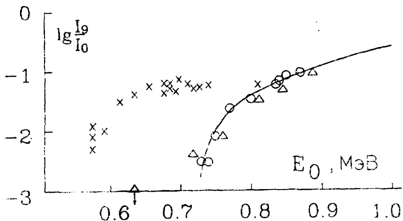
Рис. 14. Зависимость ослабления тока электронов I_0/I_0 алюминиевой фольгой толщиной l=1310 мкм от исходной энергии E_0 . Сплошная линия — расчет по К. Эксперимент: \circ — измерения в диоде (N1329), \Delta — на выходе соленоида при n_0 = 2 \cdot 10^{16} \text{ см}^{-3} (N1259), \times — на выходе соленоида при n_0 = 7 \cdot 10^{12} \text{ см}^{-3} (N1255).
