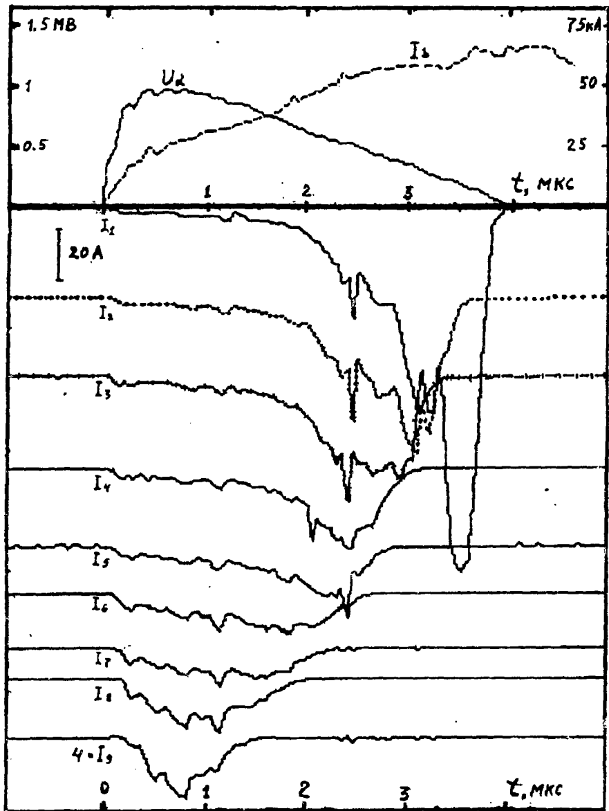
Рис. 3. Типичные осциллограммы напряжения на диоде U_d , тока пучка I_b , токов I_1 — I_9 электронов на фольге (N1329: МФА сразу за анодной фольгой); l_1 — l_5 —100, l_6 — l_7 —150, l_8 —400, l_9 —900 мкм.
