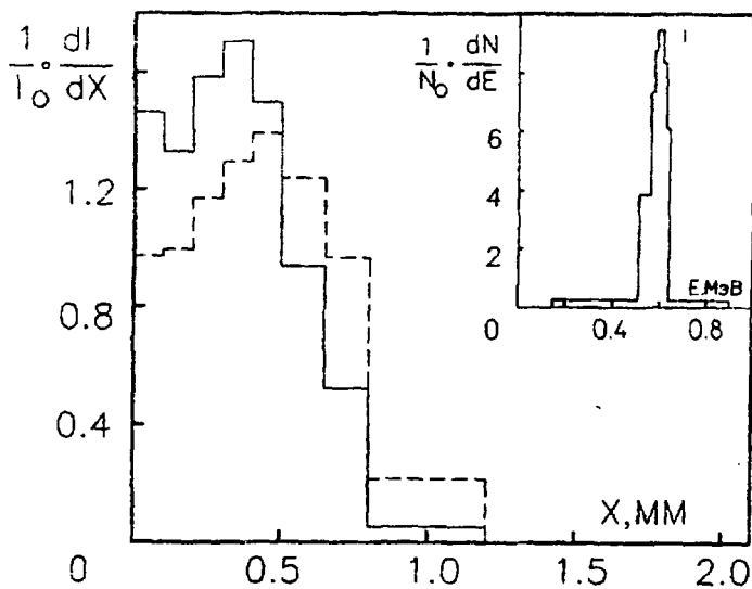
Рис. 10. Экспериментальная гистограмма токов (сплошная линия) при U_d \approx 0.7 МВ и толщине дополнительной фольги 106 мкм (N1320: МФА сразу за анодной фольгой), восстановленный по ней спектр РЭП (на врезке) и, для сравнения, экспериментальная гистограмма токов при том же напряжении без дополнительной фольги на анализаторе (N1329).
