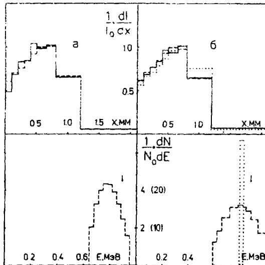
Рис. 8. Гистограммы токов (вверху) и спектры энергий (внизу) для двух последовательных выстрелов (а—N1328, б — N1329) при одинаковом напряжении на диоде U_d = 0.87 МВ (МФА сразу за анодной фольгой). Сплошные линии—экспериментальные гистограммы. Пунктир—восстановленные по экспериментальным значениям токов спектры энергий (а - E_{cp} = 0.89eU_d , б - E_{cp} = 0.91eU_d ) и восстановленные по этим спектрам гистограммы. Точки—спектр дельта-функции (шкала 35 МэВ) и соответствующая ей гистограмма.
