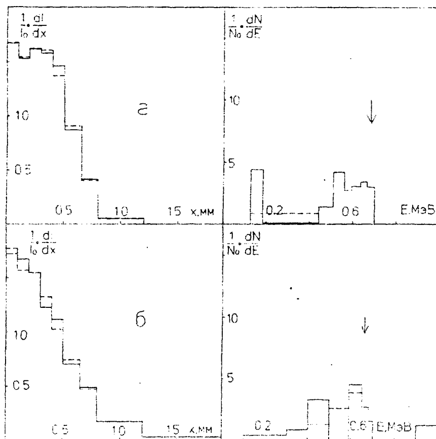
Рис. 13. Гистограммы токов и спектры энергий РЭП (МФА на выходе соленоида): а— U_d = 0.67 \text{ МВ} ; n_0 = 1.5 \cdot 10^{15} \text{ см}^{-3} — предплазма (N1264); б— U_d = 0.66 \text{ МВ} ; n_0 = 7 \cdot 10^{12} \text{ см}^{-3} (N1255).
