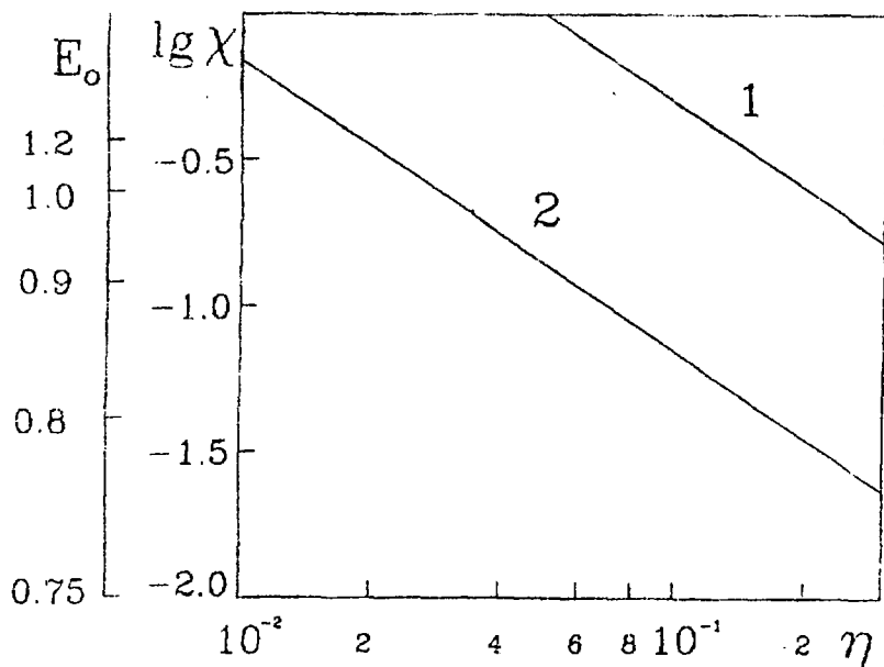
Рис. 15. Зависимость коэффициента ослабления \chi ускоренных частиц от их доли в пучке \eta : 1 — \chi \cdot \eta = 0.05 ( E = 0.65 - 0.75 МэВ); 2 — \chi \cdot \eta = 0.007 ( E = 0.57 МэВ).
