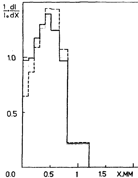
Рис. 6. Сравнение экспериментальной гистограммы тока (N1329) U_d = 0.7 МВ—(сплошные линии) с расчетными для дельтафункций по энергии ( E_b = 0.64 МэВ): пунктир—с использованием функции K , точки— K^* .
