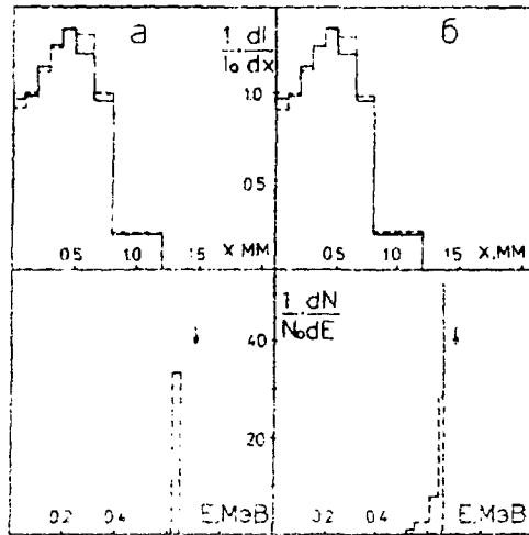
Рис. 7. Экспериментальные и расчетные гистограммы токов (вверху) и спектры энергий (внизу). Сплошные линии—экспериментальная гистограмма токов (N1329; U_d = 0.7 МВ, МФА сразу за анодной фольгой). а) Пунктир и точки - дельта-функции и рассчитанные по ним гистограммы токов. б) Пунктир—восстановленный по экспериментальным значениям токов спектр электронов и вычисленная по нему гистограмма. (Стрелками здесь и ниже на рисунках указаны значения E = eU_d .)
