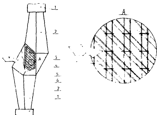
Рис. 1. Конструкция дискретного монитора: 1 - фотоумножители; 2 - воздушные световоды; 3 - лавсановые нити; 4 - рамка матрицы; 5 - пучок; 6 - сцинтилляционные палочки.
