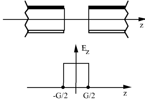
Fig. 1 RF gap
