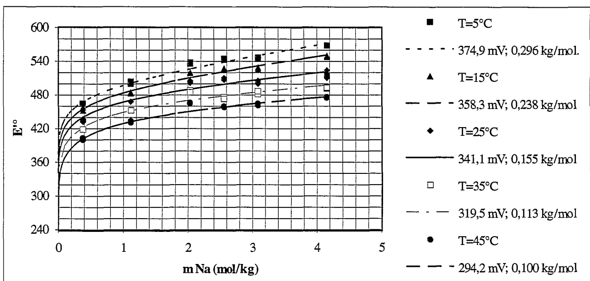
Figures A5 : Extrapolation à force ionique nulle, de potentiels d'oxydoréduction du couple Np(VI)/Np(V) mesuré en milieu \text{Na}_2\text{CO}_3 . E^\circ est en mV/ENH, A = R T \ln(10) / F vaut 59,16 mV à 25°C (annexe A3), m\text{Na} est la molalité de \text{Na}^+ . Les droites de régression utilisant la formule de la TIS, sont tracées avec les valeurs indiquées dans la légende. D est le terme de Debye-Hückel, les figures 4 sont des extraits de ces figures GRAFEX.XLS
