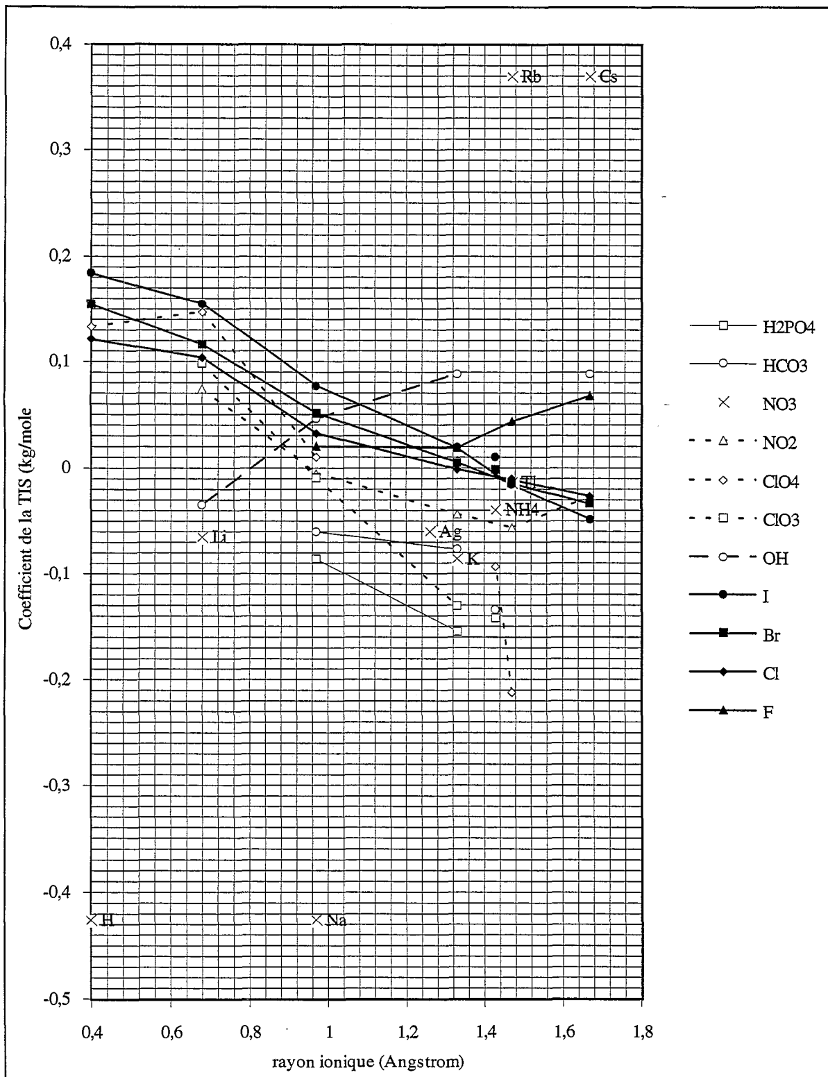
Figure S3.1.d : corrélation entre \epsilon et rayon ionique, voir les légendes des figures S3.1.
