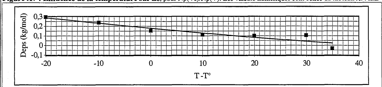
Figure A7 : Influence de la température sur \Delta\epsilon , pour Np(VI)/Np(V). Les valeurs numériques sont celles du tableau A7 . DE.XLS
