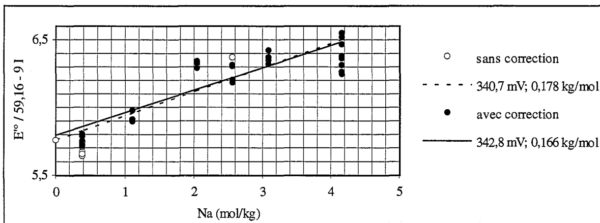
Figure A10 : Correction de la dissociation du complexe limite de Np(V). Les droites de régression de la TIS, sont tracées avec les valeurs de E^\circ(25^\circ\text{C}, 0) (mV/ESH) et \Delta \varepsilon(25^\circ\text{C}) (kg/mol.) indiquées sur la figure. FORCE.XLS
