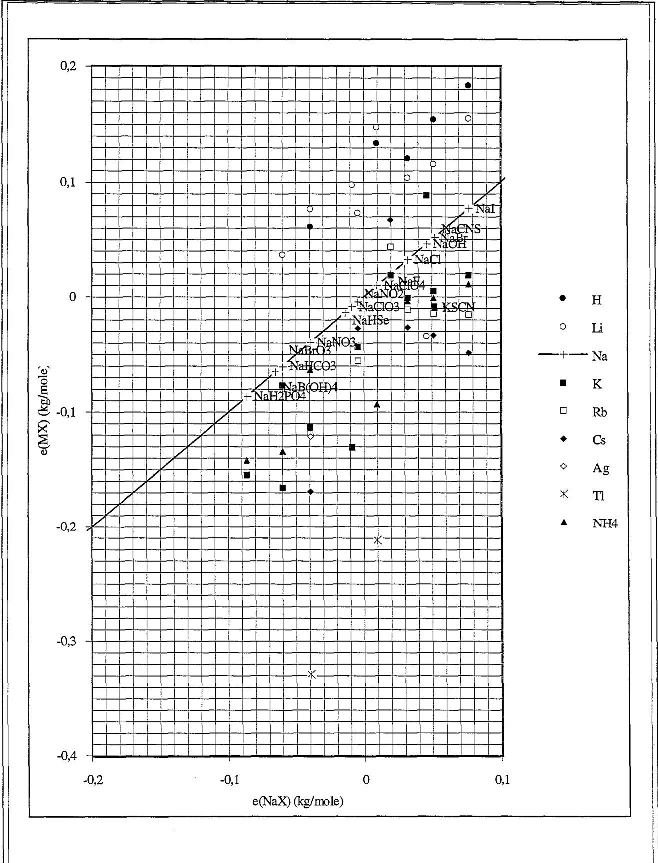
Figure S3.1.c : corrélation entre \varepsilon , détail de la figure S3.1.b.
