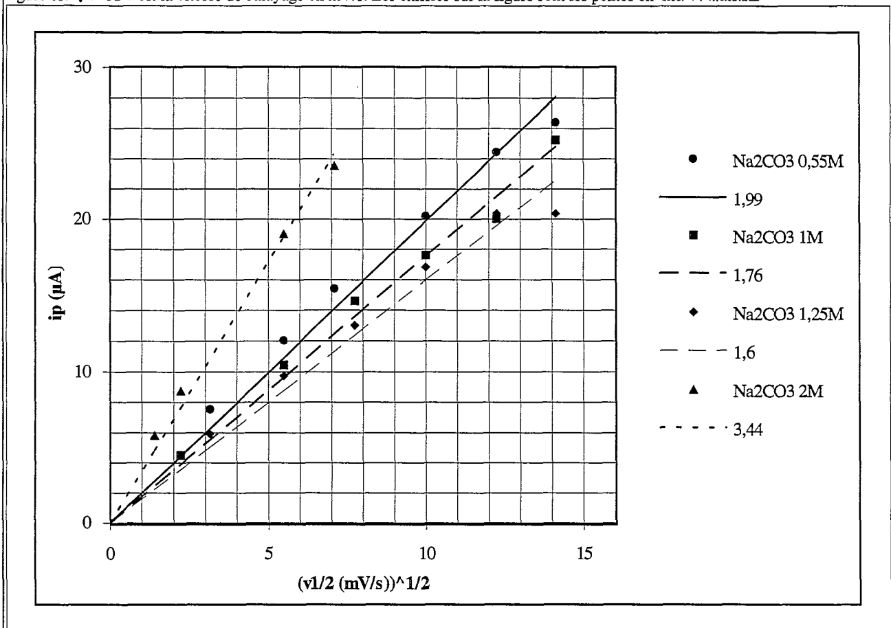
Figure 2 : Influence de la vitesse de balayage sur le courant de pic, i_p (noté i_p sur la figure). On vérifie la linéarité de i_p = f(\sqrt{v}) . i_p est ici le pic d'oxydation. T = 25^\circ\text{C} , les points expérimentaux sont ceux de l'annexe 2, v^{1/2} ( \text{mV/s} ) 1/2 noté sur la figure est \sqrt{v} où v est la vitesse de balayage en \text{mV/s} . Les chiffres sur la figure sont les pentes en \text{mc/V} . VITGRAPH.XLS
