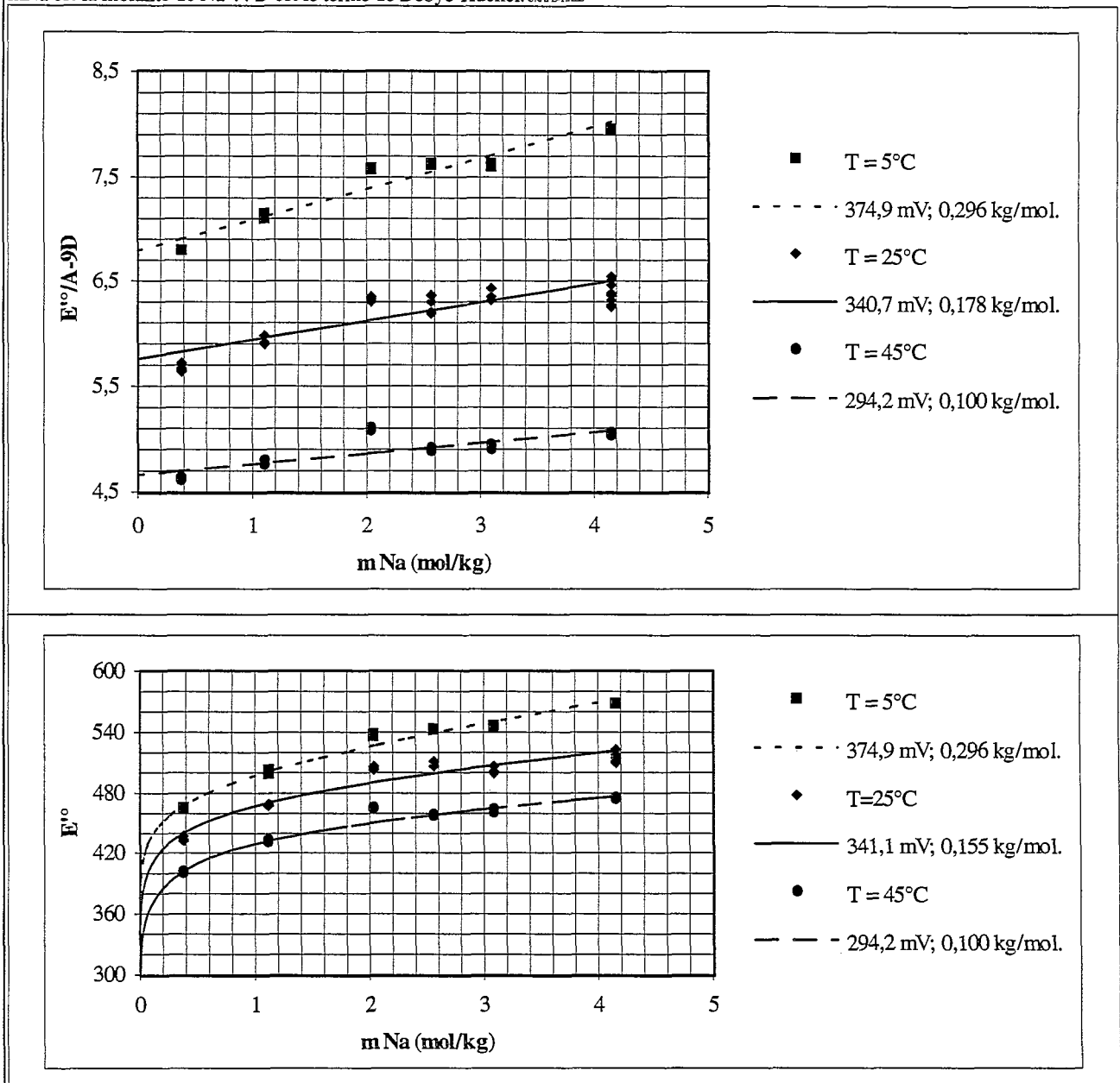
Figure 4 : Extrapolation à force ionique nulle, du potentiel d'oxydoréduction du couple Np(VI)/Np(V) mesuré en milieu \text{Na}_2\text{CO}_3 . Le potentiel mesuré, E^\circ (mV/ENH), est extrapolé à I=0 selon la formule (4-10) de la TIS. Les droites de régression, sont tracées avec les valeurs indiquées dans la légende : E^\circ à I=0 (mV/ENH) et \Delta\varepsilon (kg/mol.). A=R T \ln(10) / F , A=59,16 mV à 25^\circ\text{C} , m\text{Na} est la molalité de \text{Na}^+ . D est le terme de Debye-Hückel. GRAPE-T.XLS
