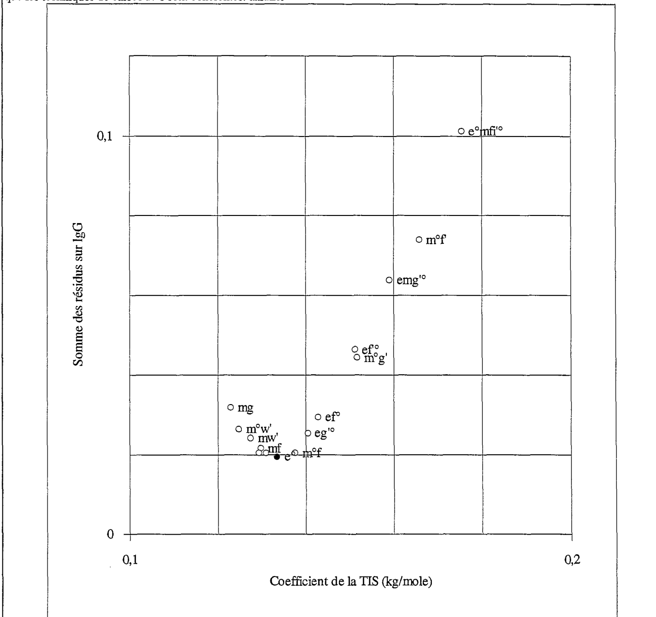
Figure S2.2.d : calcul de \varepsilon(\text{H}^+, \text{ClO}_4^-) . Cette figure est analogue à la figure S2.2.c , elle permet de vérifier sur un électrolyte fort, que les techniques de calcul de \varepsilon sont cohérentes. GHCL0A.DOC
