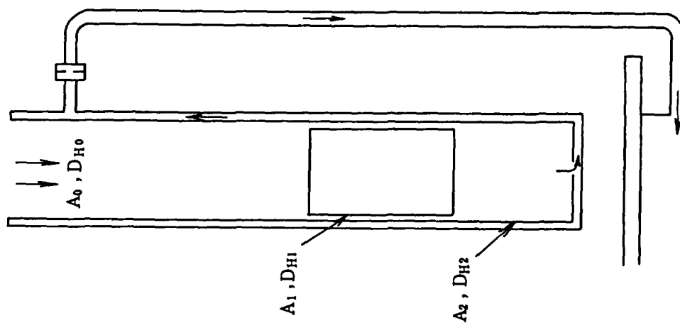
Fig. B-10 照射サンプル SH (照射物冷却管付)
