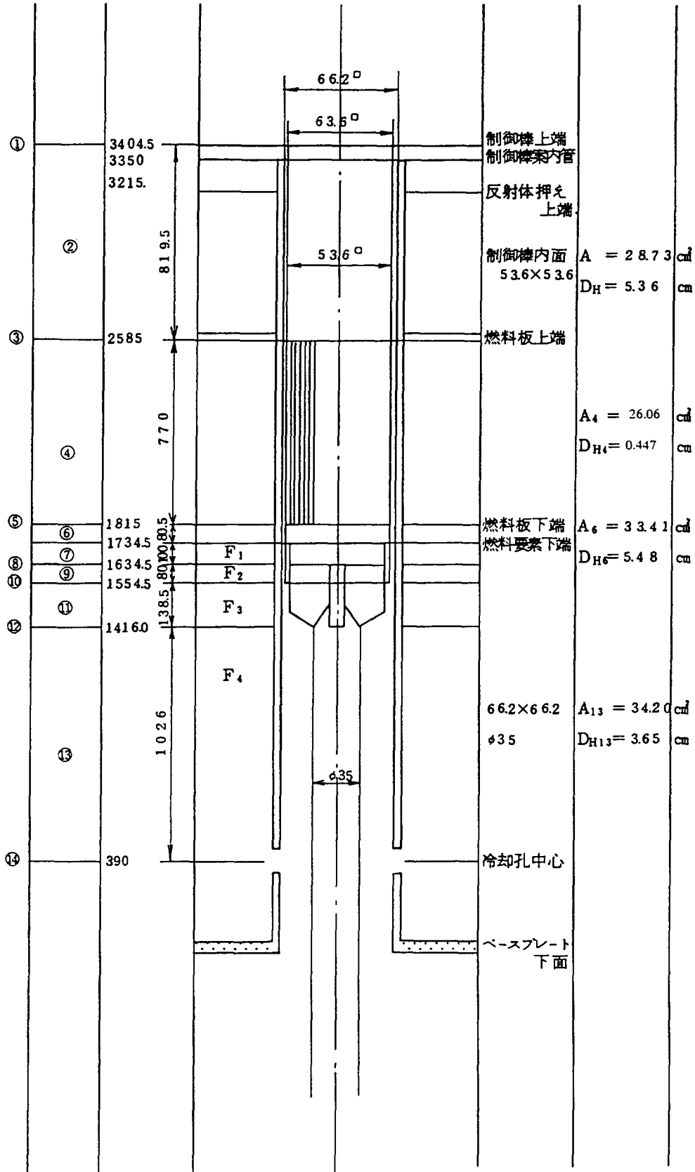
Fig. B-2 フォロワ型燃料要素の軸方向領域分割
