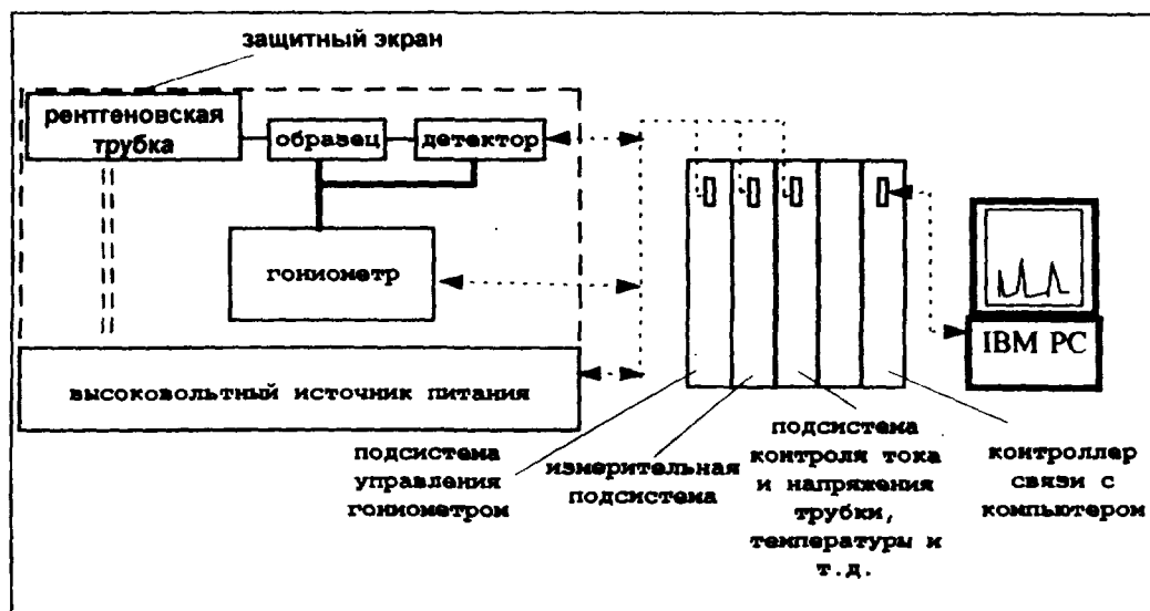
Рис. 1 Рентгеновская установка ДРОН-2-М
