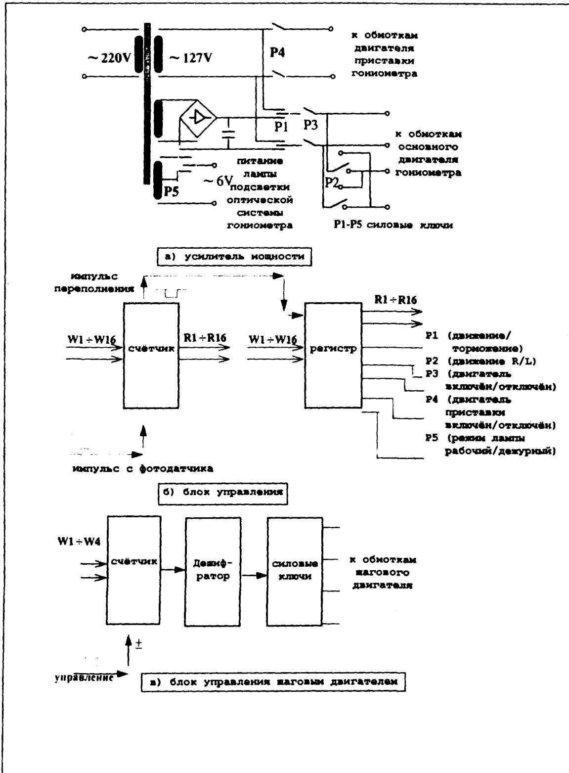
Рис. 2 Организация управления гониометром
