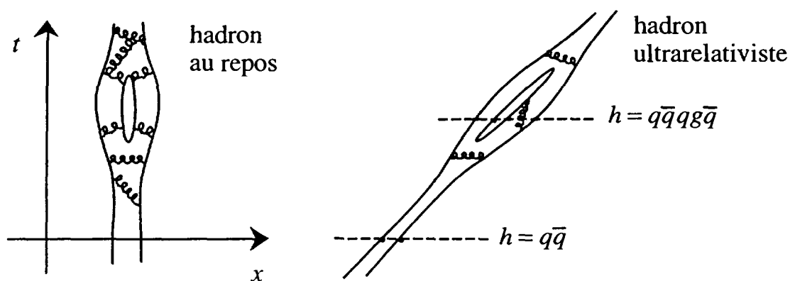
figure représentant l'évolution temporelle d'un hadron.
