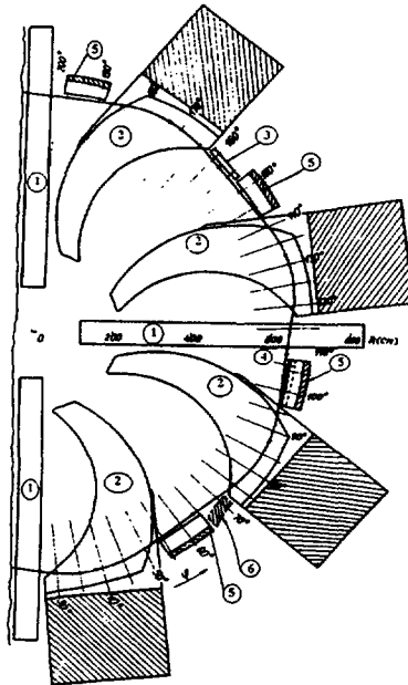
Рис. 2. Схема ускорителя проекта "Суперциклотрон". 1 - резонаторы, 2 - секторные магниты, 3,4,5,6 - элементы системы вывода
