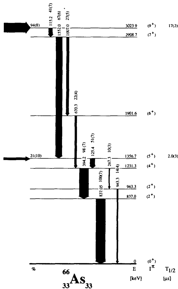
Figure 2 : schéma de décroissance des deux états isomériques observés de ^{66}\text{As} . L'intensité des transitions est proportionnelle à la largeur des flèches correspondantes.
