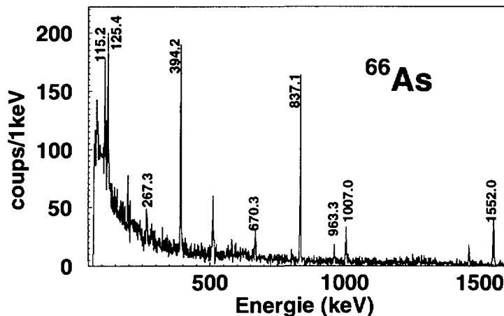
Figure 1 : spectre en énergie des \gamma détectés dans un délai de 50 \mu\text{s} après l'implantation d'un ion ^{66}\text{As} .
