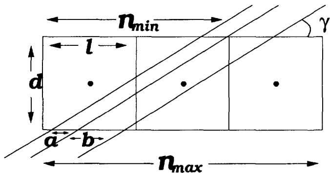
Рис. 1: Проекция трека на плоскость, перпендикулярную всем сигнальным проводочкам
